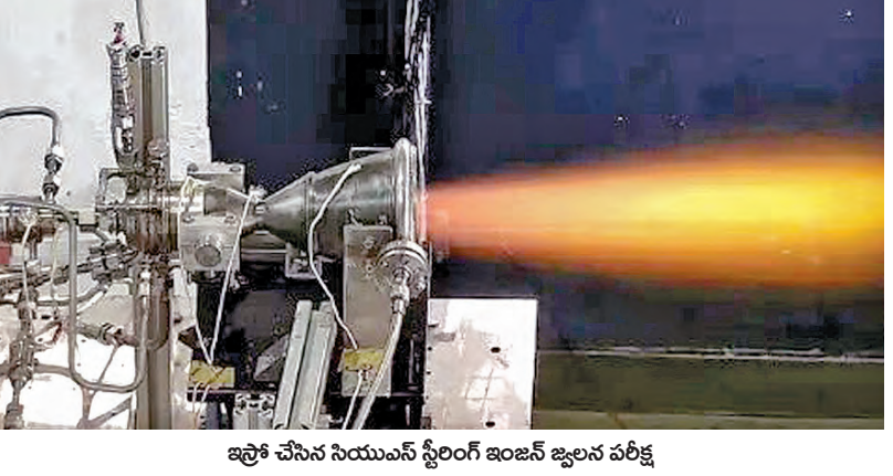
ఇల్వో చేసిన సి ఎంఎస్ స్పిరింగ్ ఇంజన్ జ్వలన పరీక్ష
