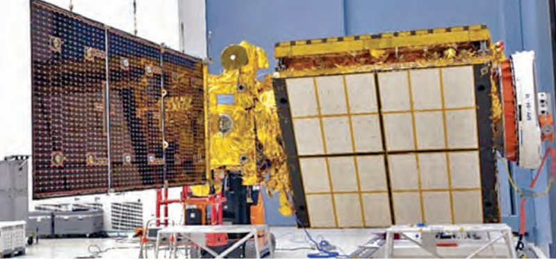
జనవరి09 ఉపగ్రహం సోలార్ ప్యానెళ్లు
