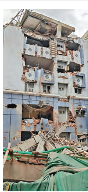
గచ్చిబౌలిలో కూలిన భవనం
